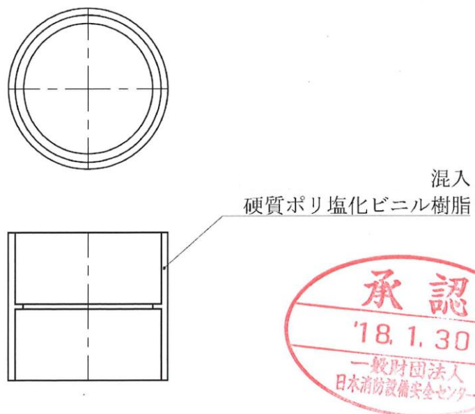
混入硬質ポリ塩化ビニル管継手の断面構造例
