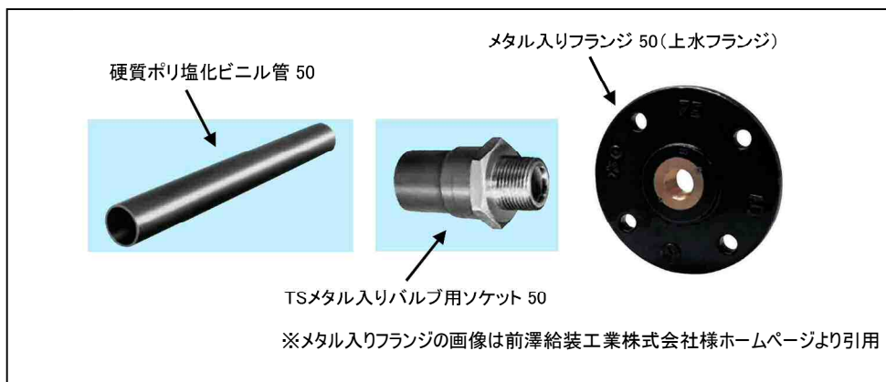
図-3.水道メーター50mm 上水フランジとの接続方法(例)
