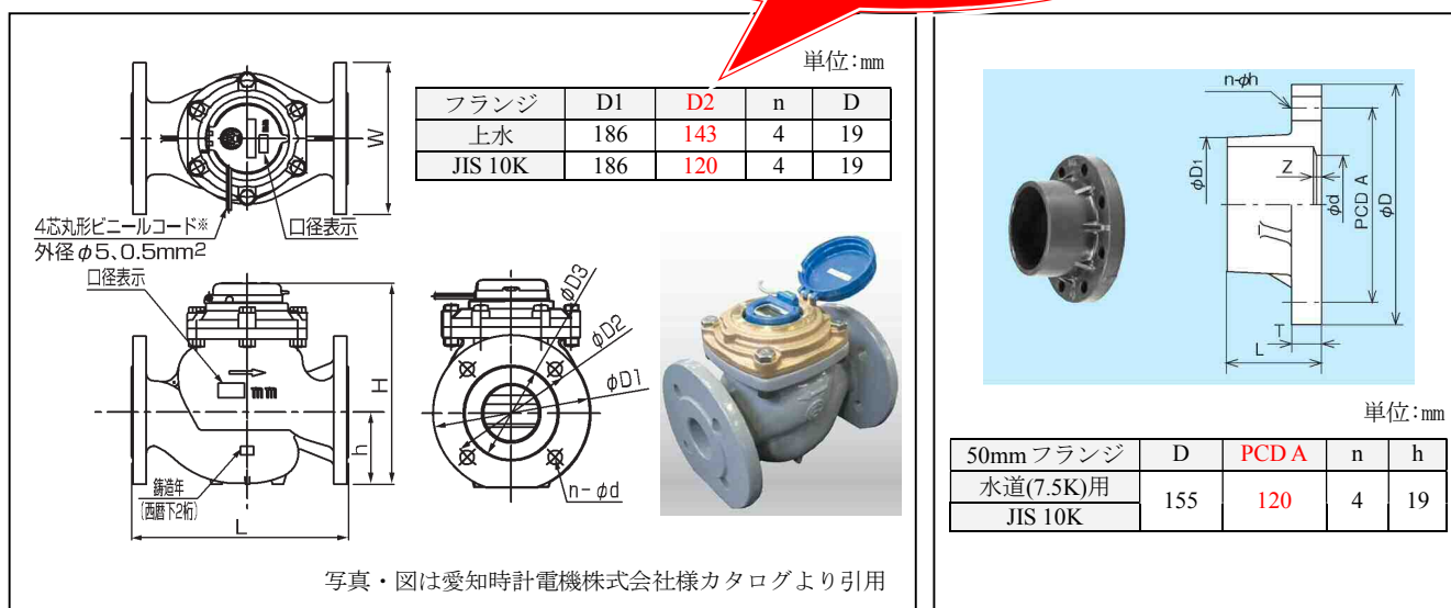
図-1. 水道メーター50mm の形状寸法
