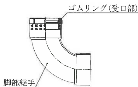
脚部継手①(代表例)
