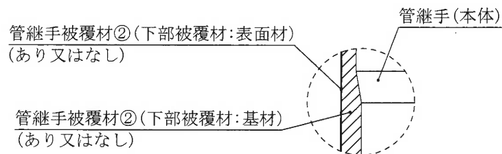
E 部詳細図
