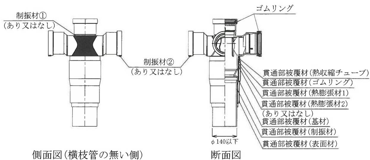
管継手(代表例)
