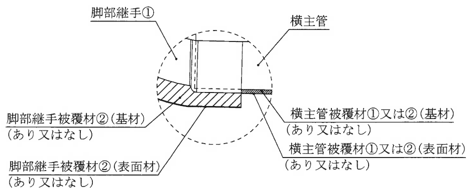
F 部詳細図
