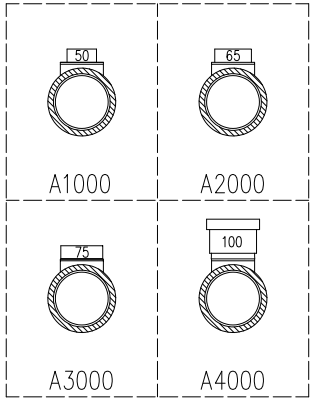
枝管バリエーション
