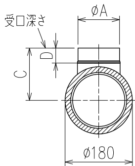
X-X断面矢視
