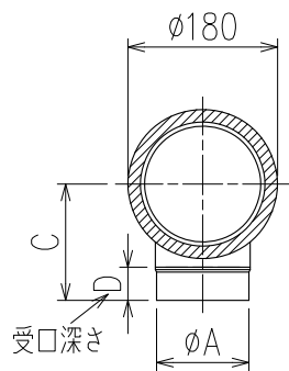
X-X断面矢視
