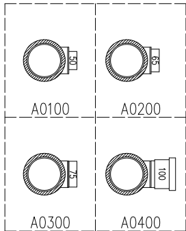
下部枝管バリエーション
