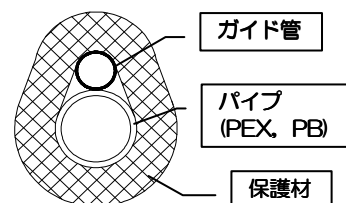
製品断面図
