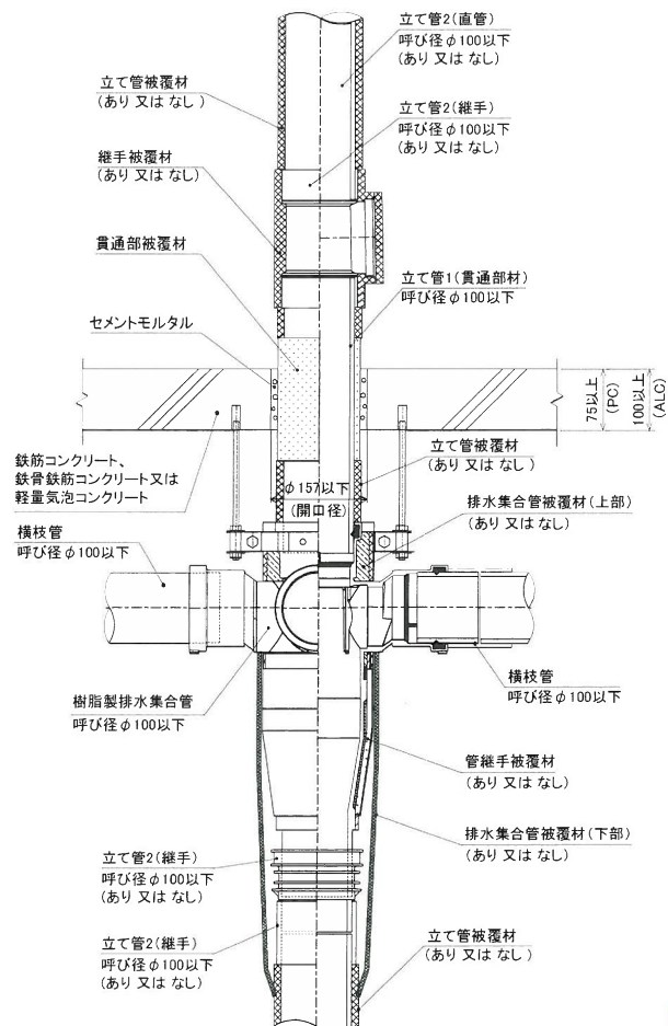
図 2 区画貫通部の断面図 (樹脂製排水集合管 代表例)
