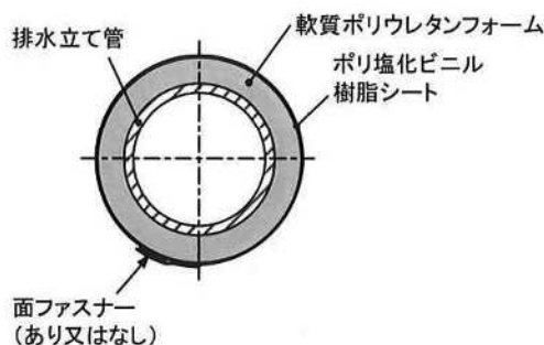
図4 被覆材①の断面図
