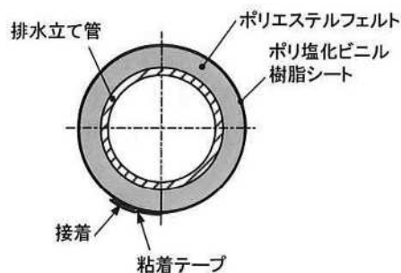
図6 被覆材②の断面図
