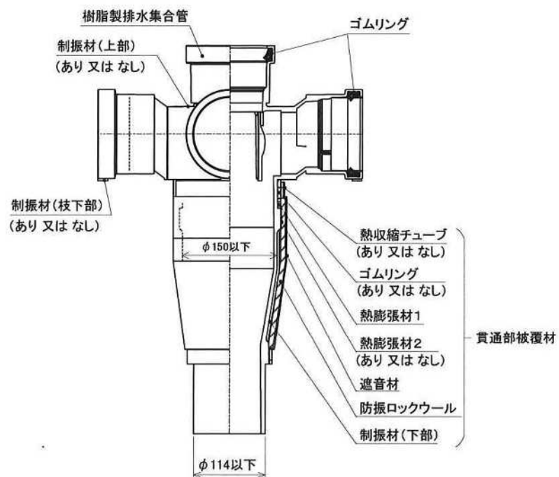
図3 樹脂製排水集合管本体の構造(代表例)
