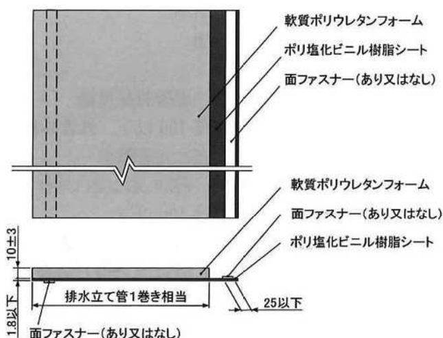
図5 被覆材①の構造
