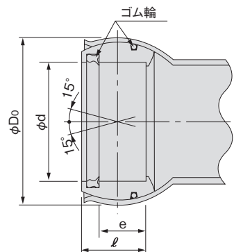
自在受口(取付け管ゴム輪受口)<支管・取付け管用> 呼び径 100~200mm
