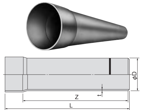
接着受口片受け直管
