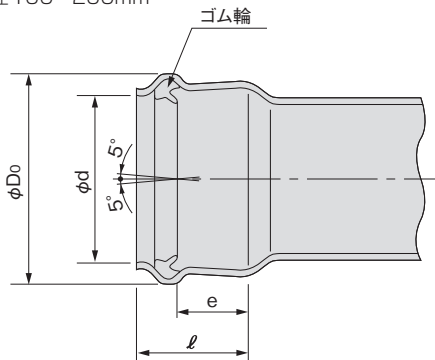
取付け管ゴム輪受口<支管・取付け管用> 呼び径 100~200mm
