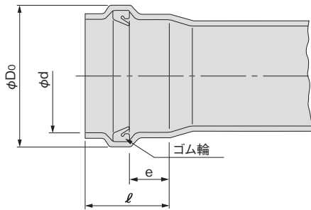
本管ゴム輪受口<本管用> 呼び径 100~600mm
