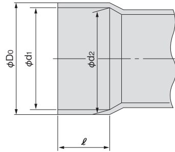
接着受口<本管・取付け管用> 呼び径 100~600mm
