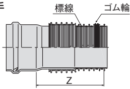
VU-RR受口-リブ差し口変換継手
