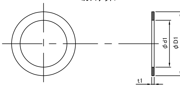
〈ガスケット〉
