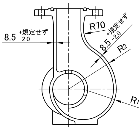
A-A 矢視図
