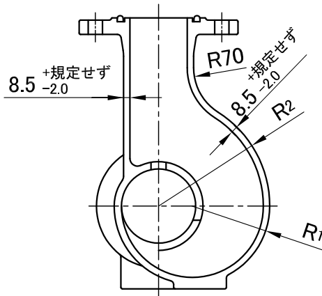
A-A 矢視図
