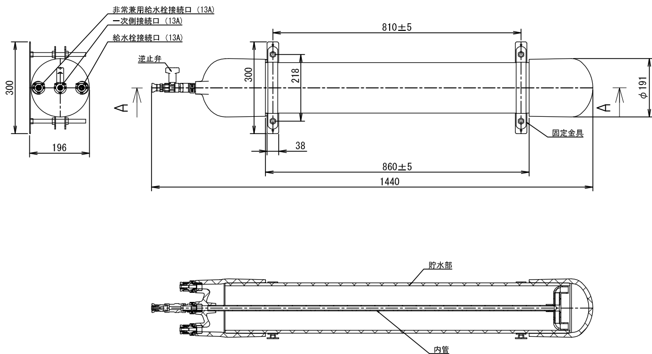
断面図 A-A
