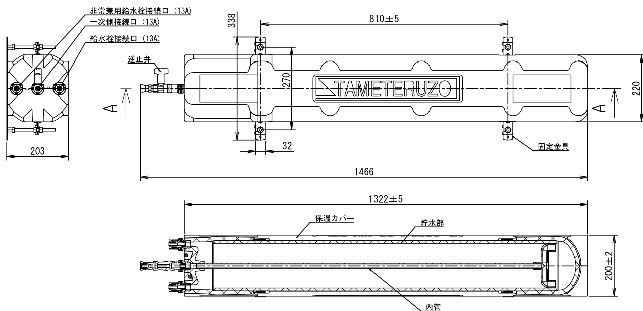
断面図 A-A
