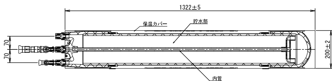
断面図 A-A
