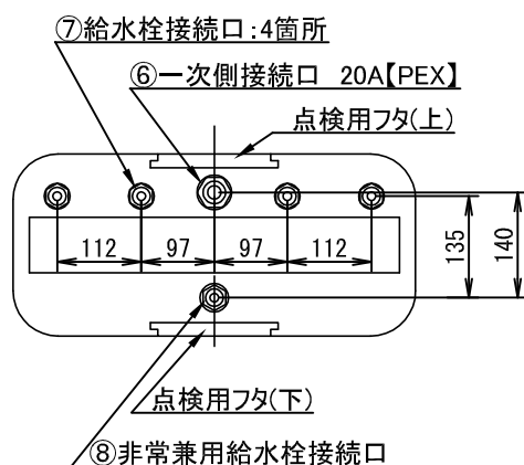
A部矢視
