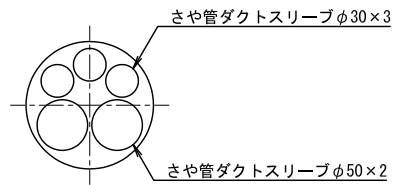
さや管ダクトスリーブ収容状態
