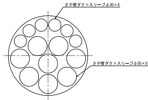
さや管ダクトスリーブ収容状態
