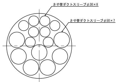
さや管ダクトスリーブ収容状態
