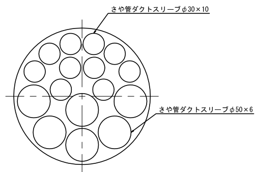
さや管ダクトスリーブ収容状態
