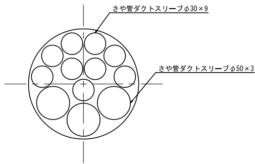
さや管ダクトスリーブ収容状態
