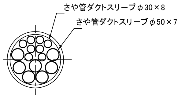
さや管ダクトスリーブ收容状態
