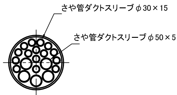
さや管ダクトスリーブ収容状態
