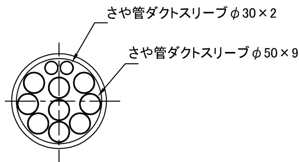
さや管ダクトスリーブ收容状態
