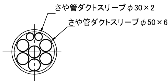
さや管ダクトスリーブ収容状態
