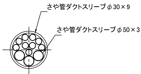
さや管ダクトスリーブ収容状態
