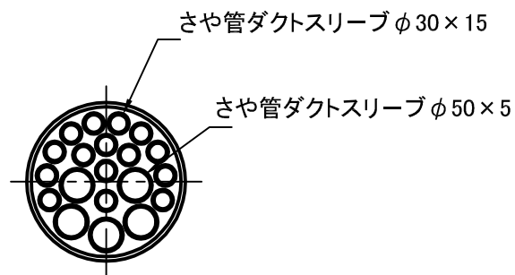
さや管ダクトスリーブ收容状態
