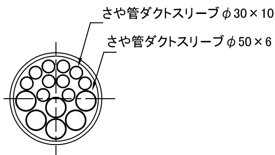
さや管ダクトスリーブ収容状態
