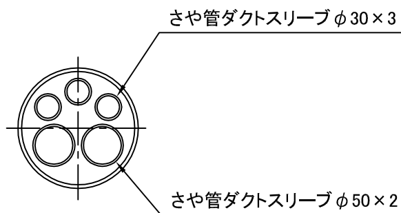
さや管ダクトスリーブ収容状態
