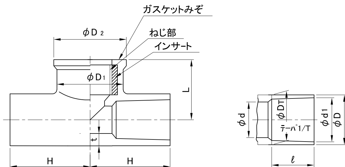
TS接合部
