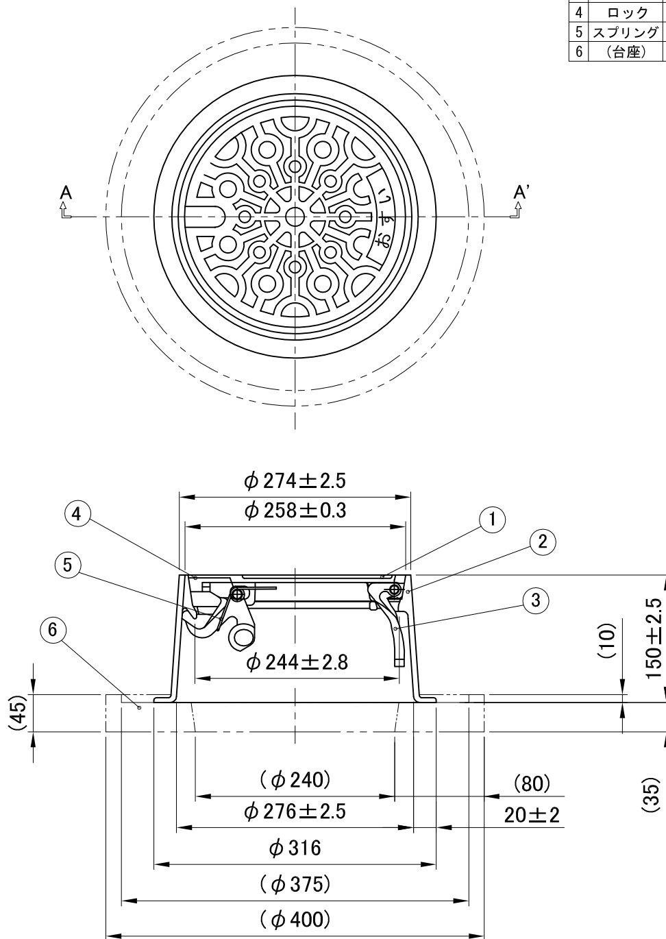
A-A'断面
