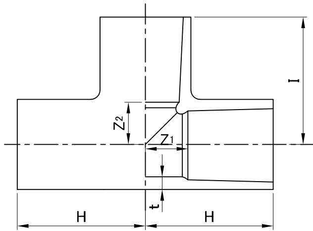
TS接合部共通寸法
