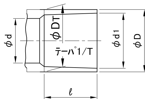
TS接合部
