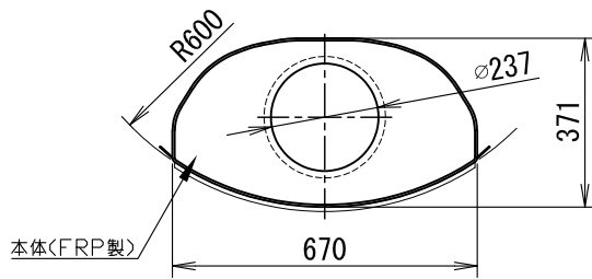
(1) 円形人孔用
