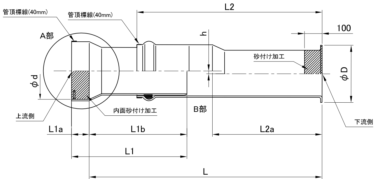
A部詳細
