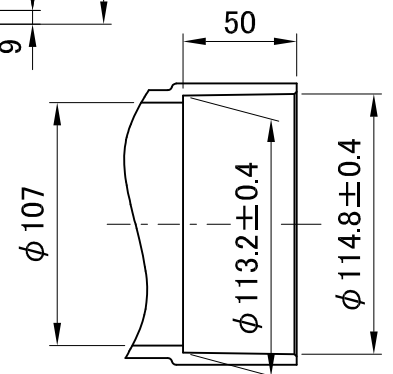
キャップ挿入部受口寸法図
