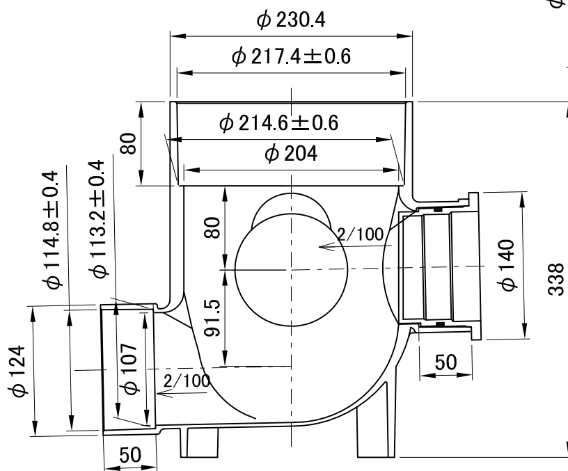
キャップ挿入部受口寸法図
