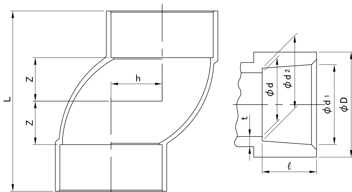
接合部共通図
