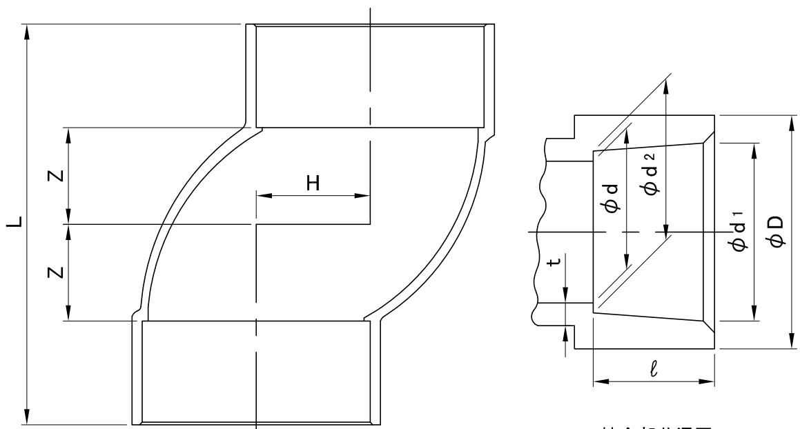
接合部共通図
