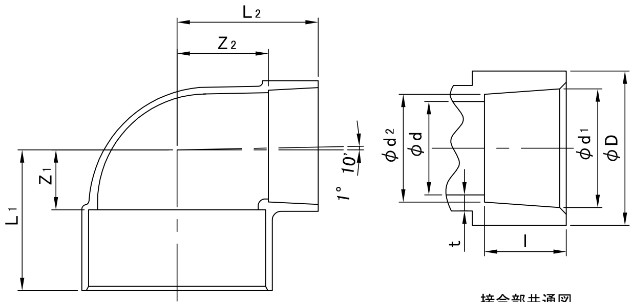
接合部共通図
