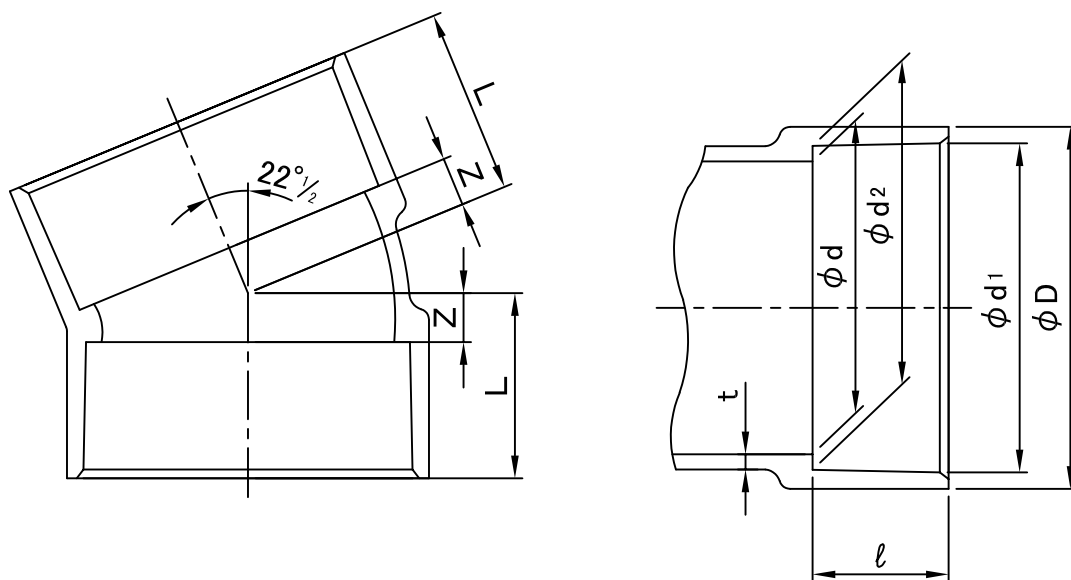
接合部共通図
