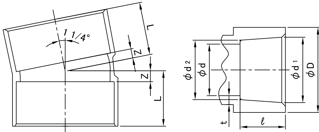
接合部共通図
