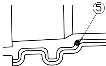
A部拡大
