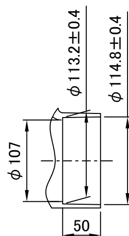
キャップ挿入部受口寸法図
