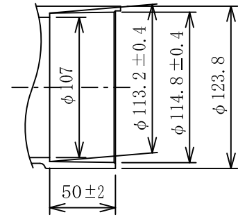
キャップ挿入部受口寸法
