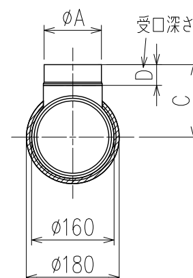
X-X断面矢視
