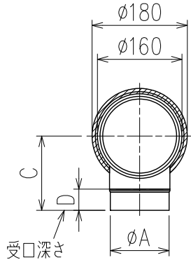
X-X断面矢視
