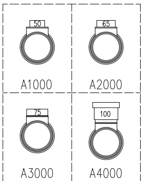
下枝管バリエーション
