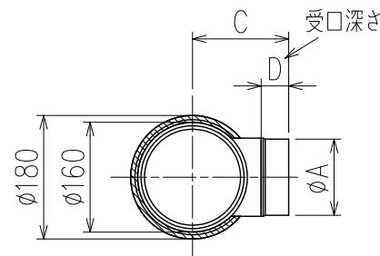
X-X断面矢視
