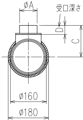
X-X断面矢視
