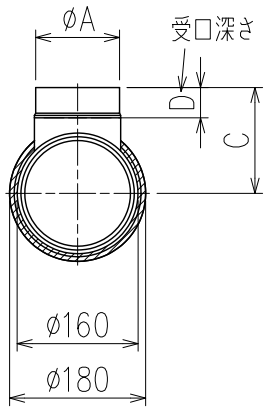
X-X断面矢視
