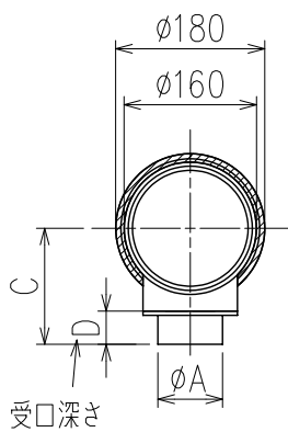
X-X断面矢視
